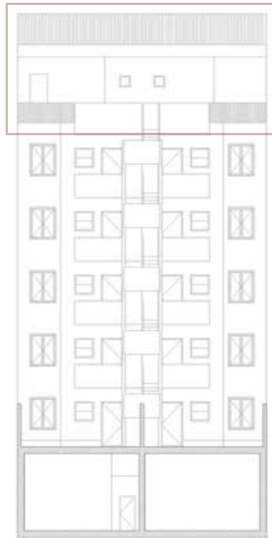
ALÇADO TARDOZ
